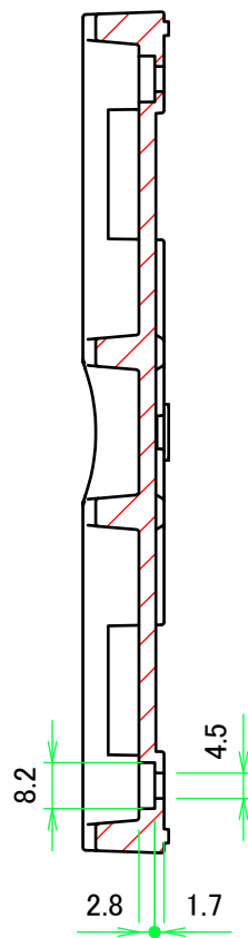
A-A (1:1.5)
